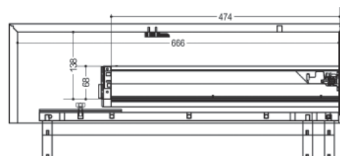
DRAWER, non-equipped
