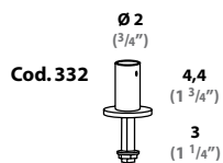
Fissaggio tavolo Cod. 332
