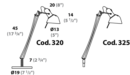
Naomi 1 Braccio Cod. 320 - 325
